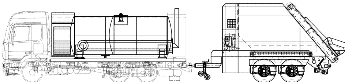
Rys. 1. Schemat kombajnu drogowego do powierzchniowego utrwalaenia nawierzchni (
